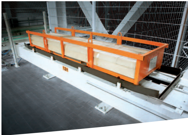
KASTO Trägerschritten mit Kundengestell.
