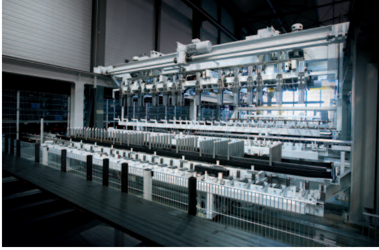
KASTO Einzelstabmanipulator mit verschiedenen Vorlagerstationen.
