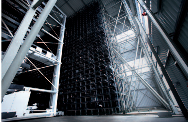
UNICOMPACT Regalblock mit Dach- und Wandanschluss.
