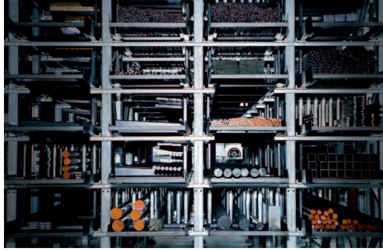
Blick in den Wabenlagerstahlbau mit Kassetten im Mischbetrieb (Automatik- und Standardkassetten).
