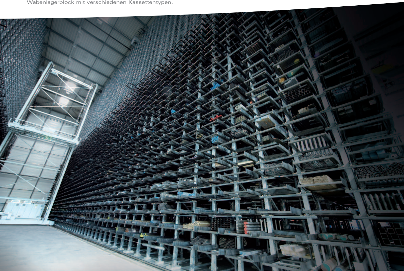
Wabenlagerblock mit verschiedenen Kassettentypen.
