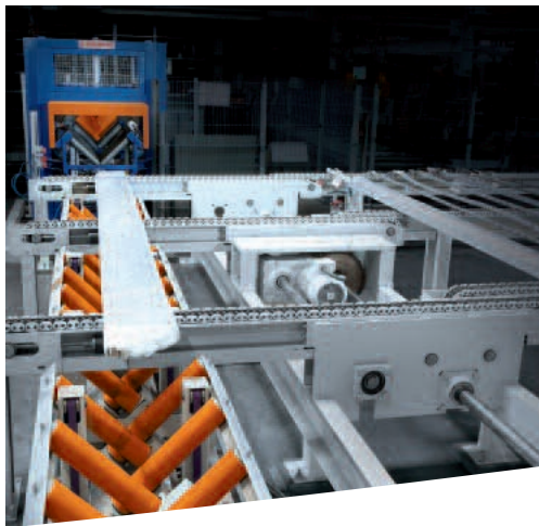
Wickelmaschine an Kommissionierstation mit heb- und senkbarer V-Rollenbahn, Stauförderer und Materialbündelförderanlage (kunststoffbelegt).
