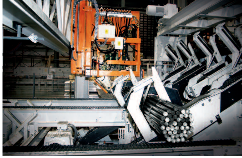
Vollautomatische Kommissionierstation mit Umreifungseinrichtung.
