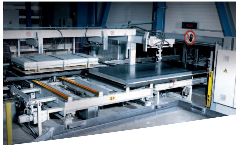
Umlaufstation mit Einlagerhilfe für Blechpakete zur Beladung mit Stapler oder Kran.
