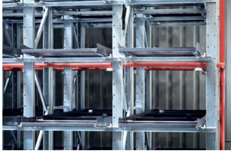
Stahlbau mit KASTO Trägerschritten und integrierter Sprinkleranlage.
