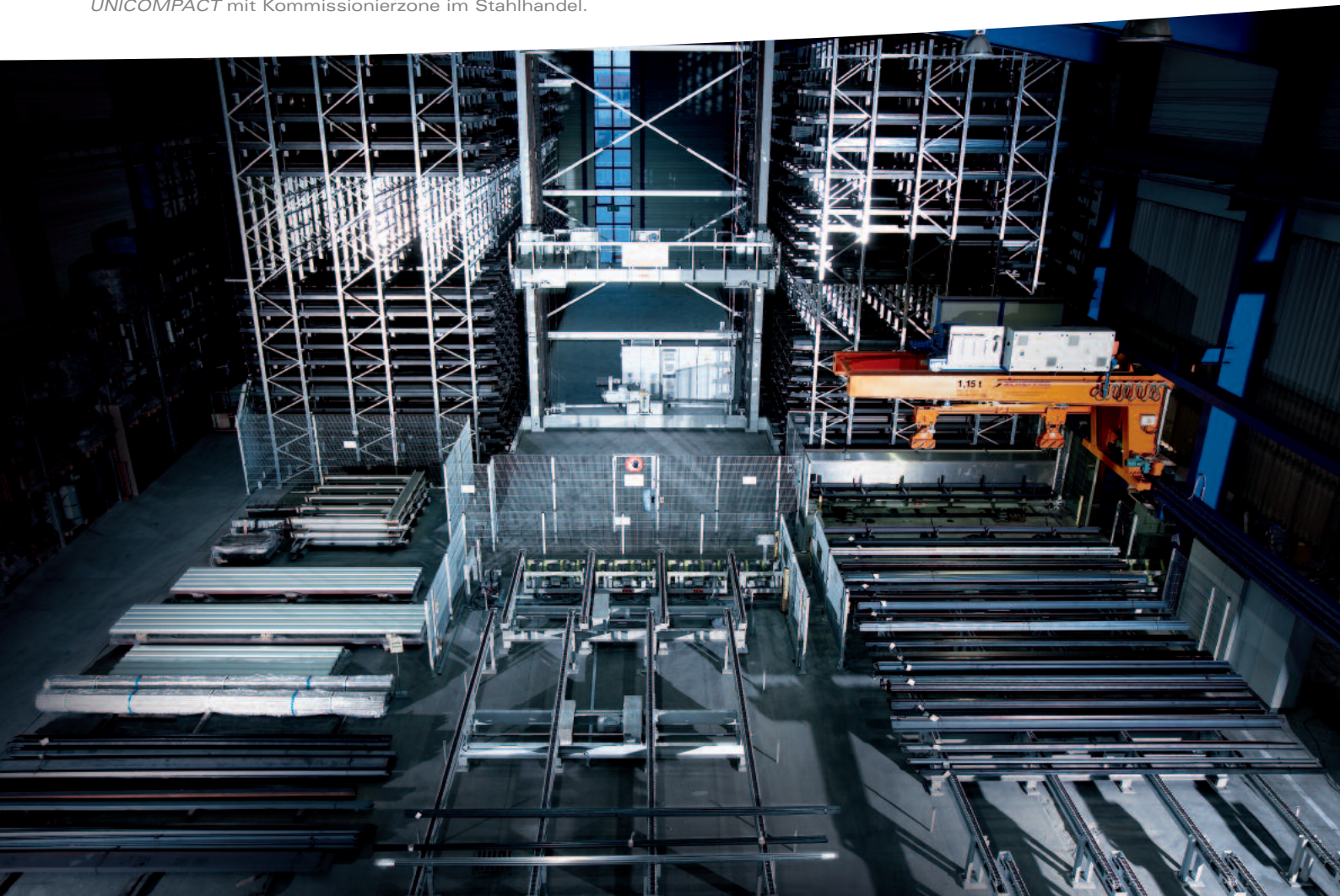
UNICOMPACT mit Kommissionierzone im Stahlhandel.
