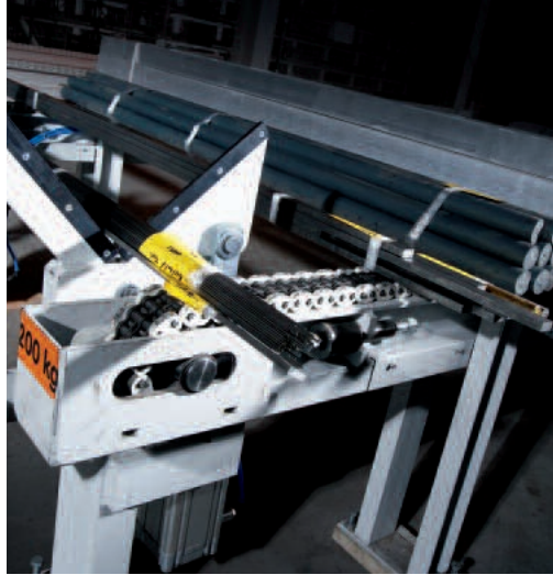
Manuelle Bündleinrichtung mit Materialbündelförderer (kunststoffbelegt).
