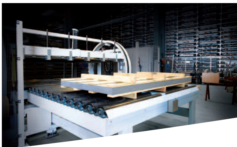
Blechwendemaschinen zum halbautomatischen Auspacken von Blechpaketen.
