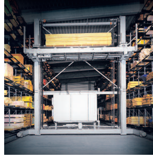
UNIGRIP im Holzhandel.
