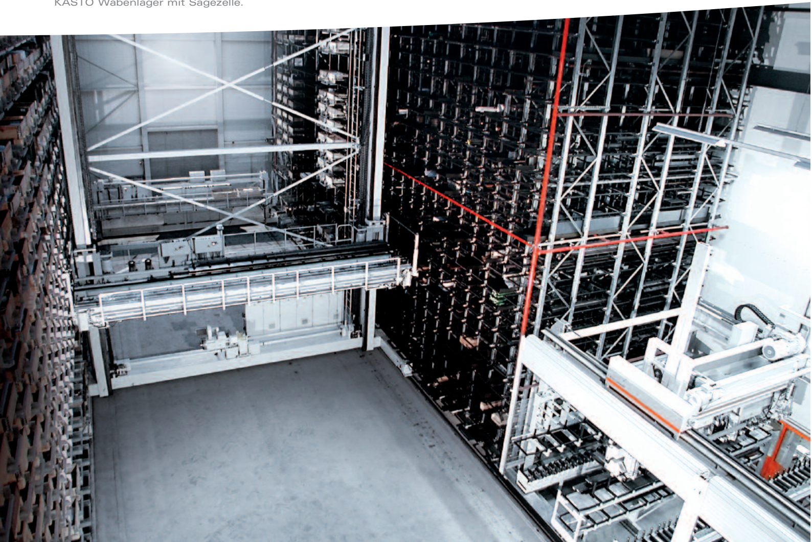
KASTO Wabenlager mit Sägezelle.
