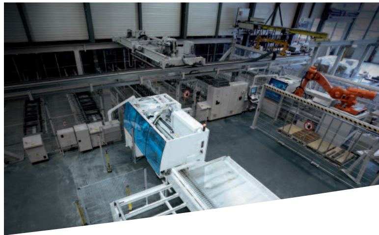
Integrierte Sägezelle KASTOsawcell an UNICOMPACT mit Direktanbindung von zwei KASTOvariospeed im Stahlhandel.
